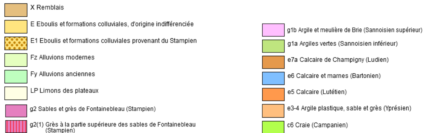
Carte géologique de Provins Source : BRGM
