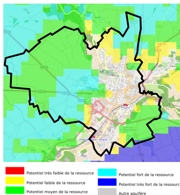
Carte du potentiel géothermique : Ressources géothermales de surface sur échangeur ouvert (nappe) en Ile de France | Source : ADEME/BRGM
