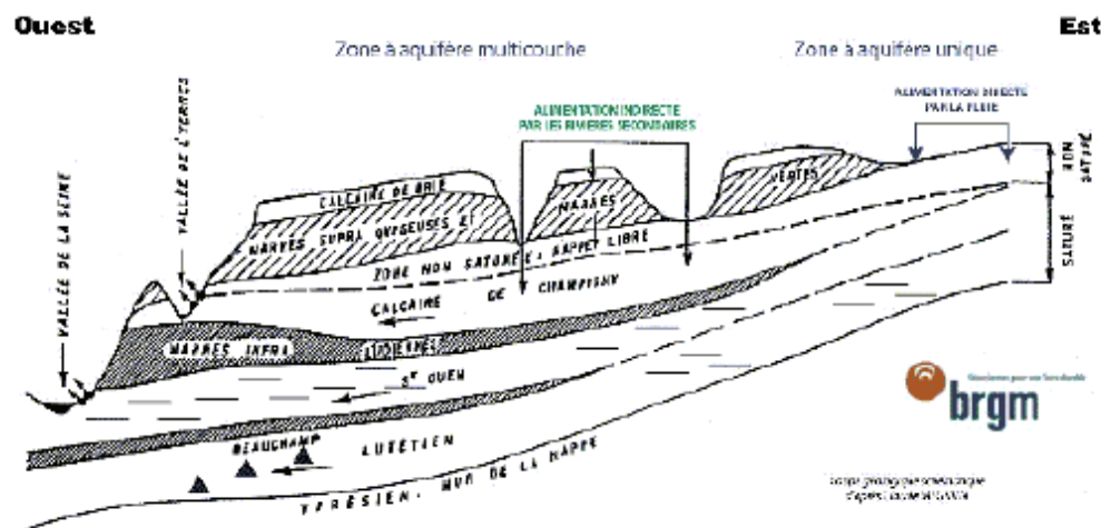
Coupe géologique Ouest-Est de la nappe des calcaires de Champigny (Source : BRGM)
